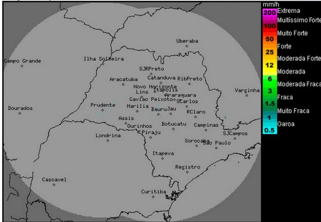
Imagem Composta dos Radares de Bauru e de Presidente Prudente - 03/06/2014 11:00
