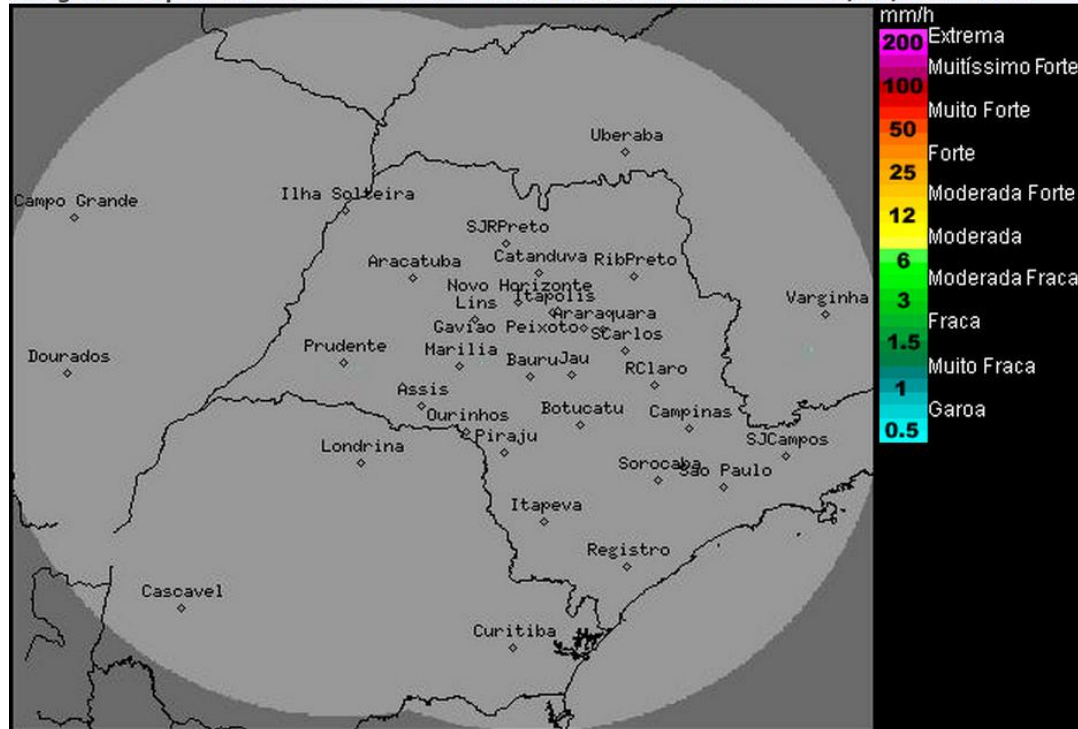
Imagem Composta dos Radares de Bauru e de Presidente Prudente - 11/05/2015 11:00
