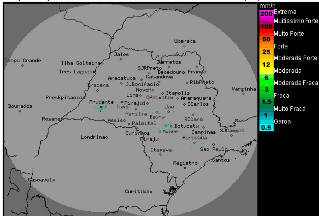
Imagem Composta dos Radares de Bauru e de Presidente Prudente - 24/11/17 08:00
