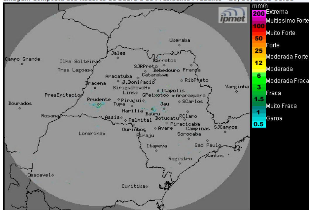
Imagem Composta dos Radares de Bauru e de Presidente Prudente - 26/06/2018 08:00
