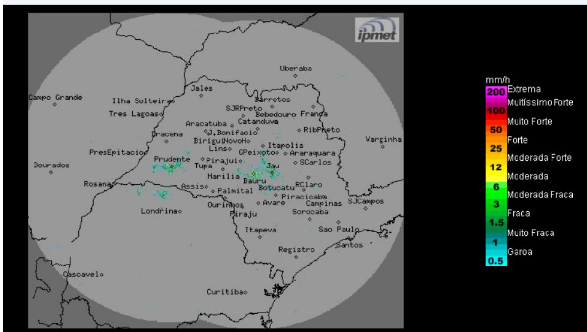
Imagem Composta dos Radares de Bauru e de Presidente Prudente - 26/07/2023 08:00
