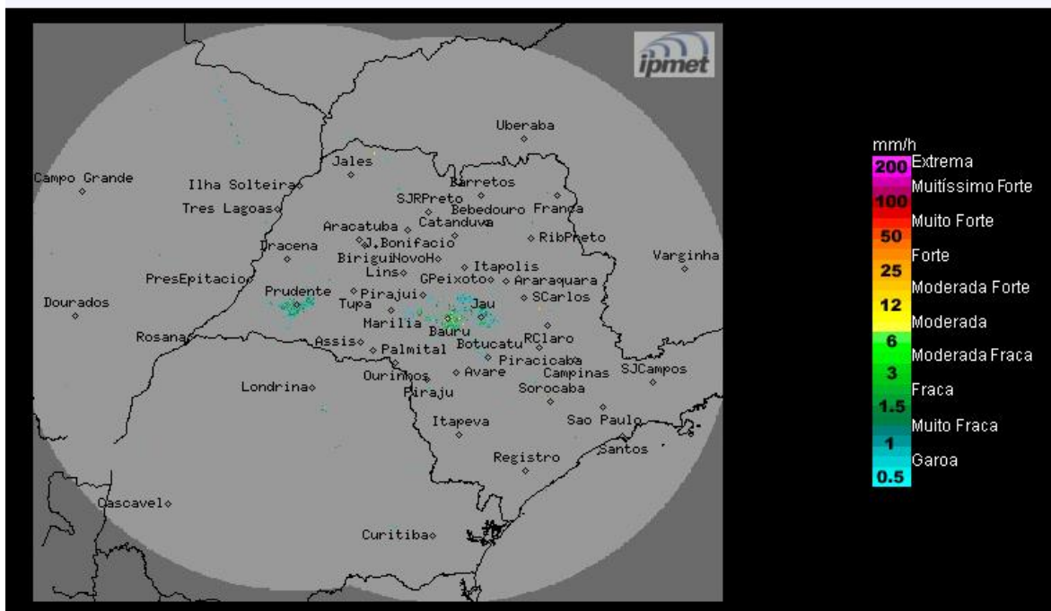
Imagem Composta dos Radares de Bauru e de Presidente Prudente - 08/05/2024 09:00
