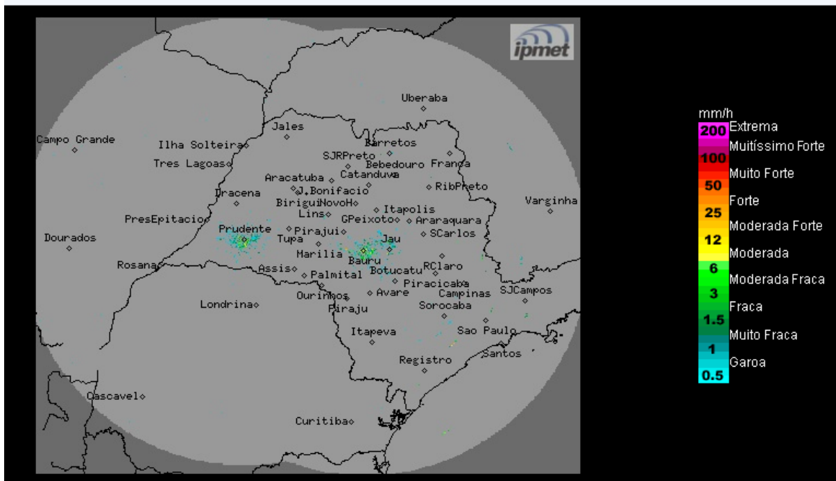
Imagem Composta dos Radares de Bauru e de Presidente Prudente - 24/12/2024 09:00
