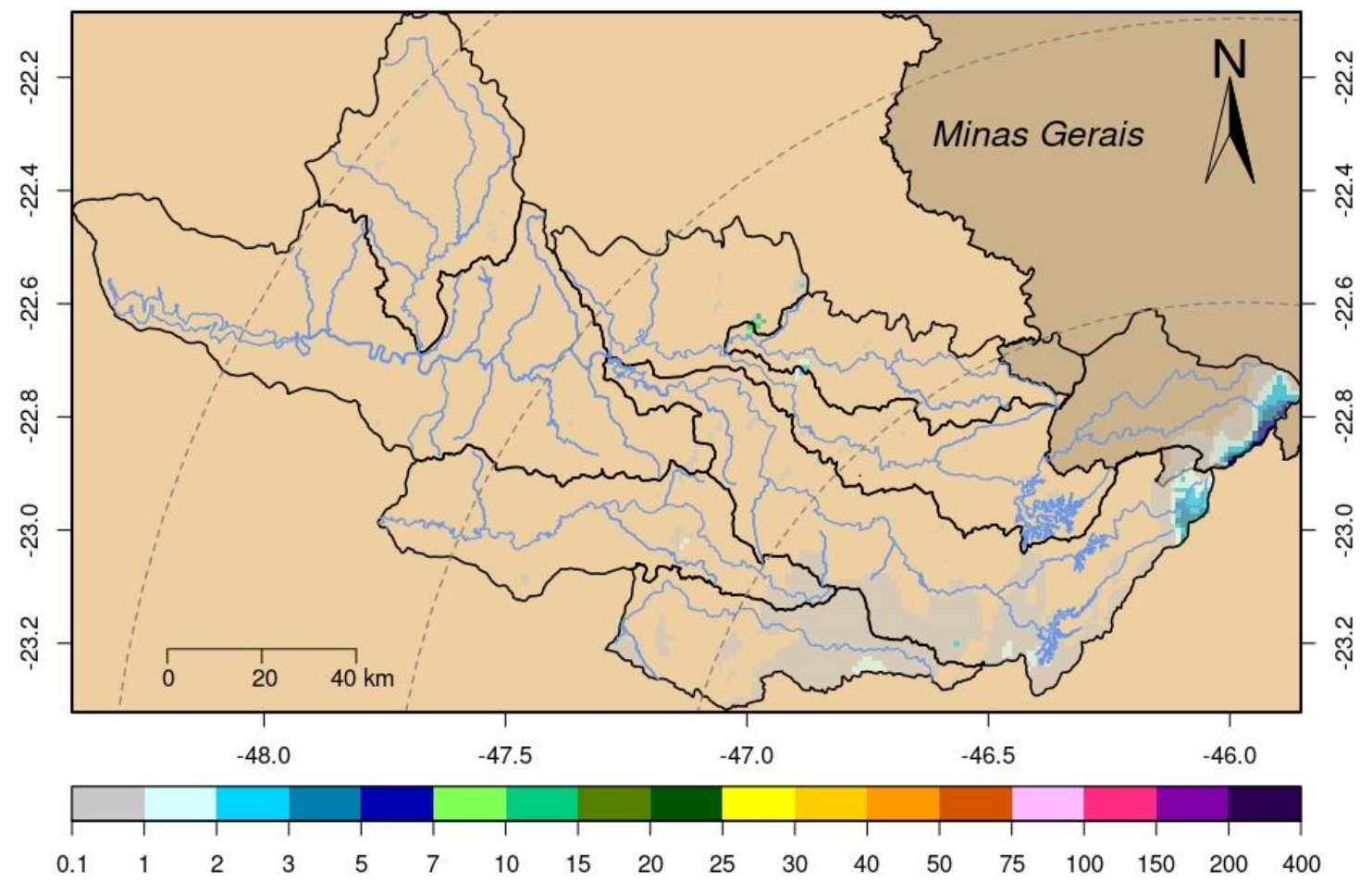
Chuva Acumulada de Radar em 24 horas nas Bacias PCJ : 24-12-2024 07:00 Local
